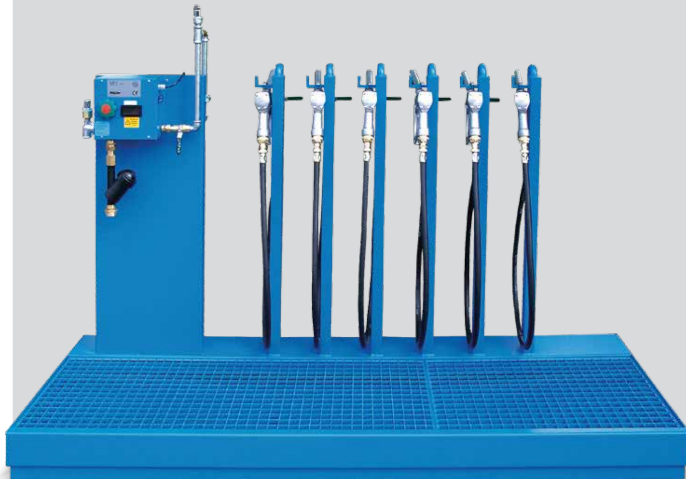
Zapfstellen für verschiedene Öle mit Mischgerät Mini digital 1500.
